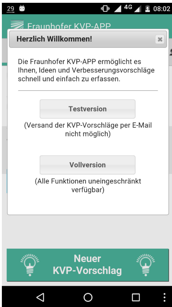
Abbildung 1: Startbildschirm
